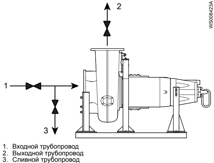
Рис. 15: Клапаны на входном, выходном и сливном трубопроводах
