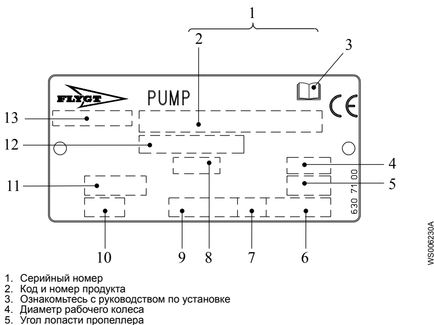
Рис. 11: Табличка для приводного блока начиная с 990101
