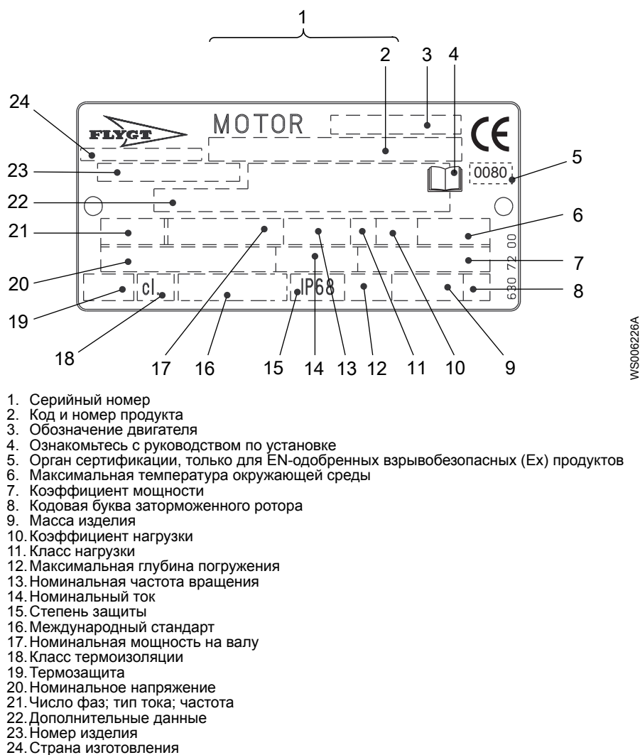
Рис. 11: Табличка для приводного блока начиная с 990101
