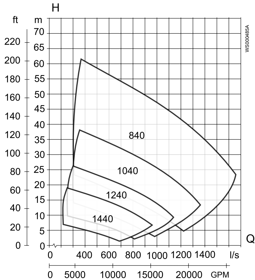
Рис. 33: C3531, 60 Hz, низкое напряжение
