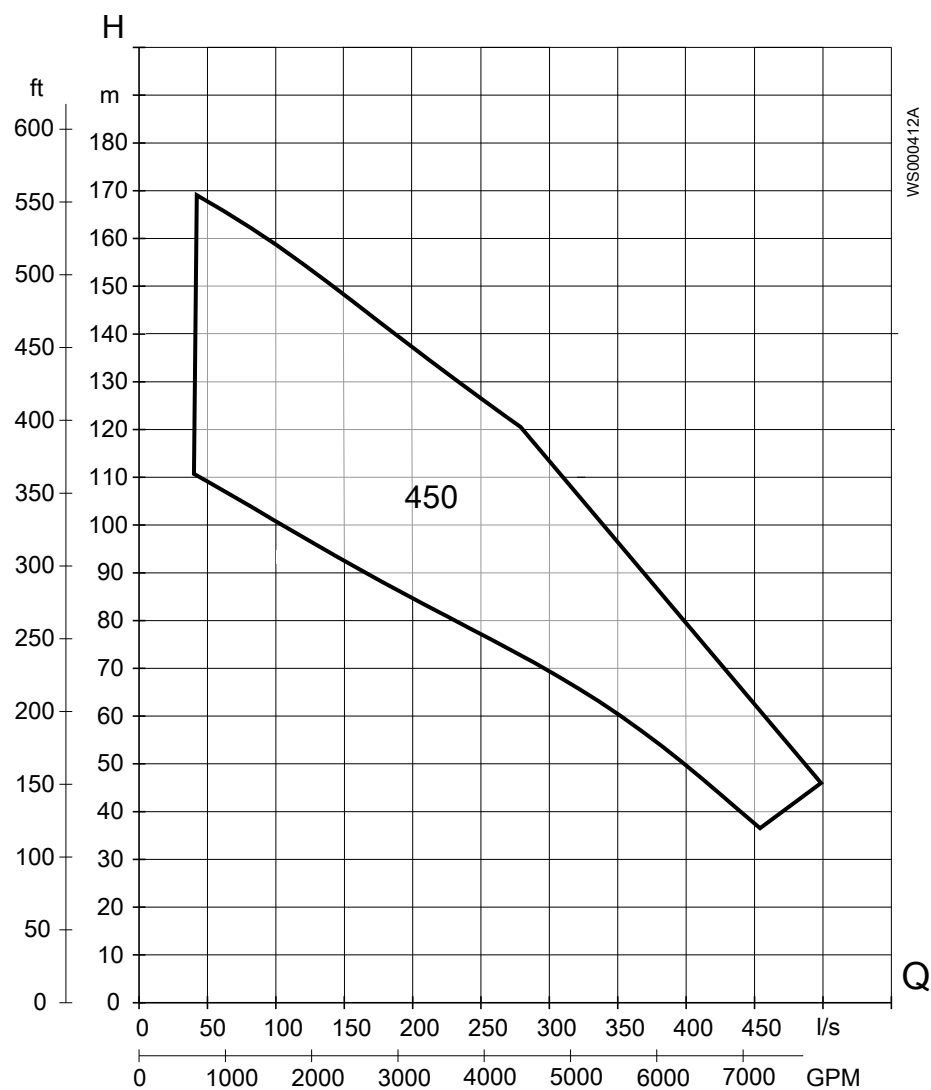
Рис. 22: C3240, 60 Hz, среднее напряжение
