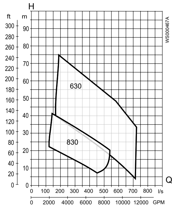
Рис. 24: С3312, 60 Hz, низкое напряжение
