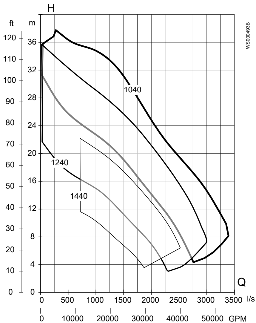
Рис. 38: C3800, 60 Hz, среднее напряжение
