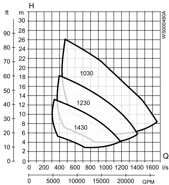
Рис. 31: C3501, 60 Hz, низкое напряжение
