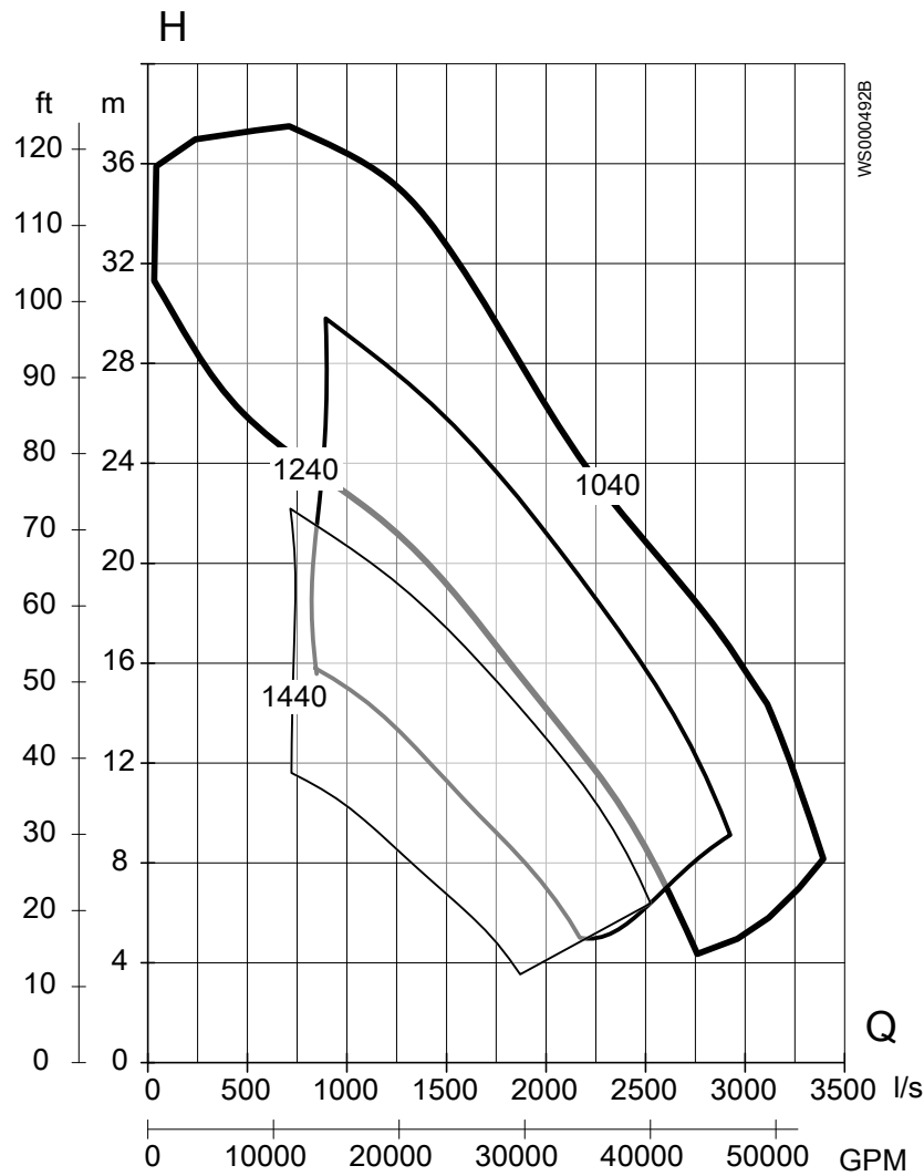
Рис. 37: C3800, 60 Hz, низкое напряжение
