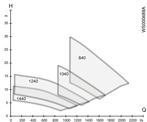
Рис. 17: С3602, 50 Hz, среднее напряжение
