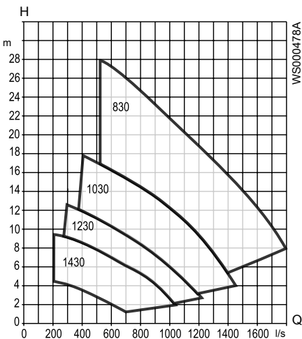
Рис. 12: С3501, 50 Hz, низкое напряжение
