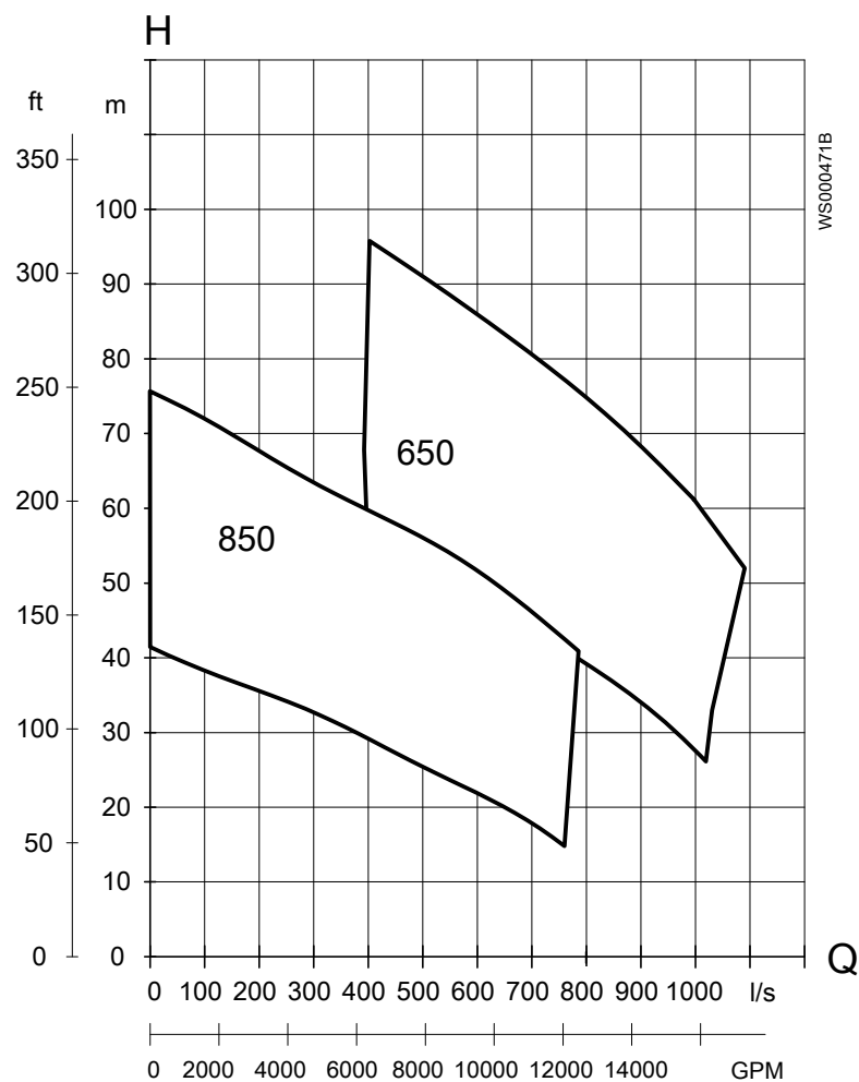
Рис. 26: C3351, 60 Hz, низкое напряжение
