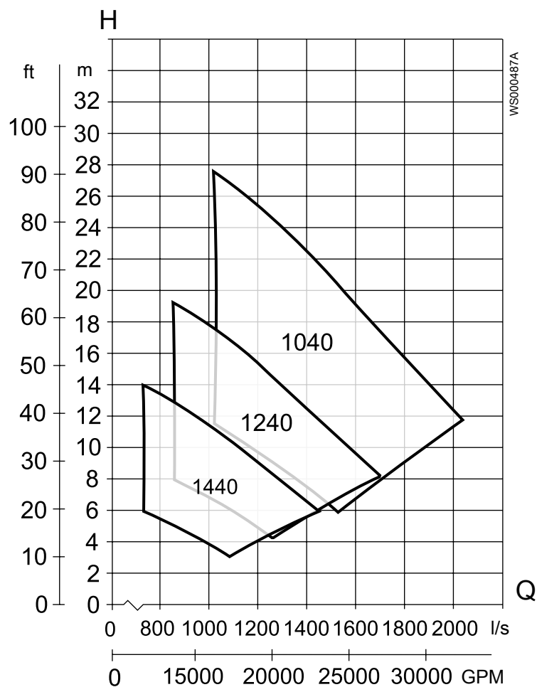
Рис. 36: C3602, 60 Hz, среднее напряжение
