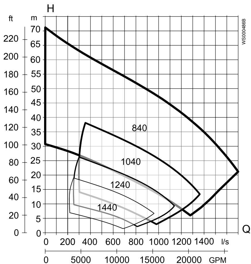
Рис. 34: C3531, 60 Hz, среднее напряжение
