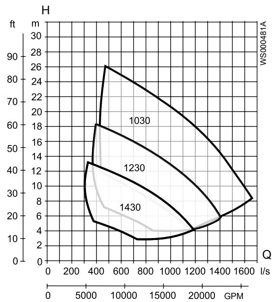
Рис. 32: C3501, 60 Hz, среднее напряжение
