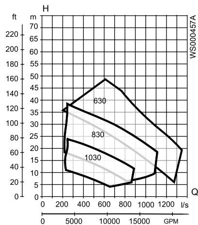
Рис. 30: C3400, 60 Hz, среднее напряжение
