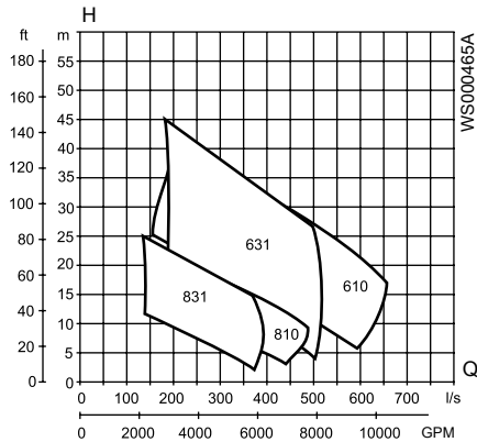
Рис. 23: C3306, 60 Hz, низкое напряжение
