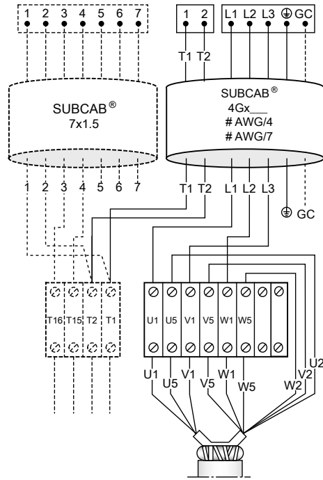
SUBCAB 4GX/SUBCAB AWG, 2 кабеля мотора, 9 выводов статора, 230 В
