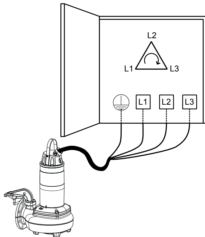
Рис. 11: Последовательность фаз
