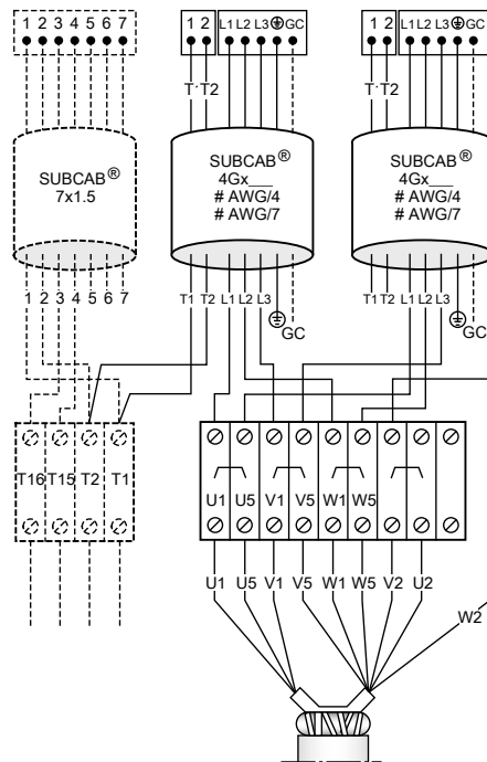
SUBCAB 4GX/SUBCAB AWG, 2 кабеля мотора, 9 выводов статора, 460 В
