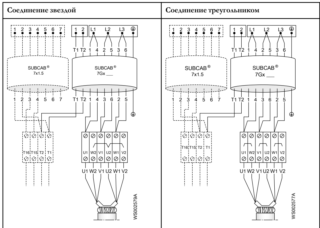
Кабель SUBCAB 7GX, 6 выводов статора, соединение звездой/треугольником
