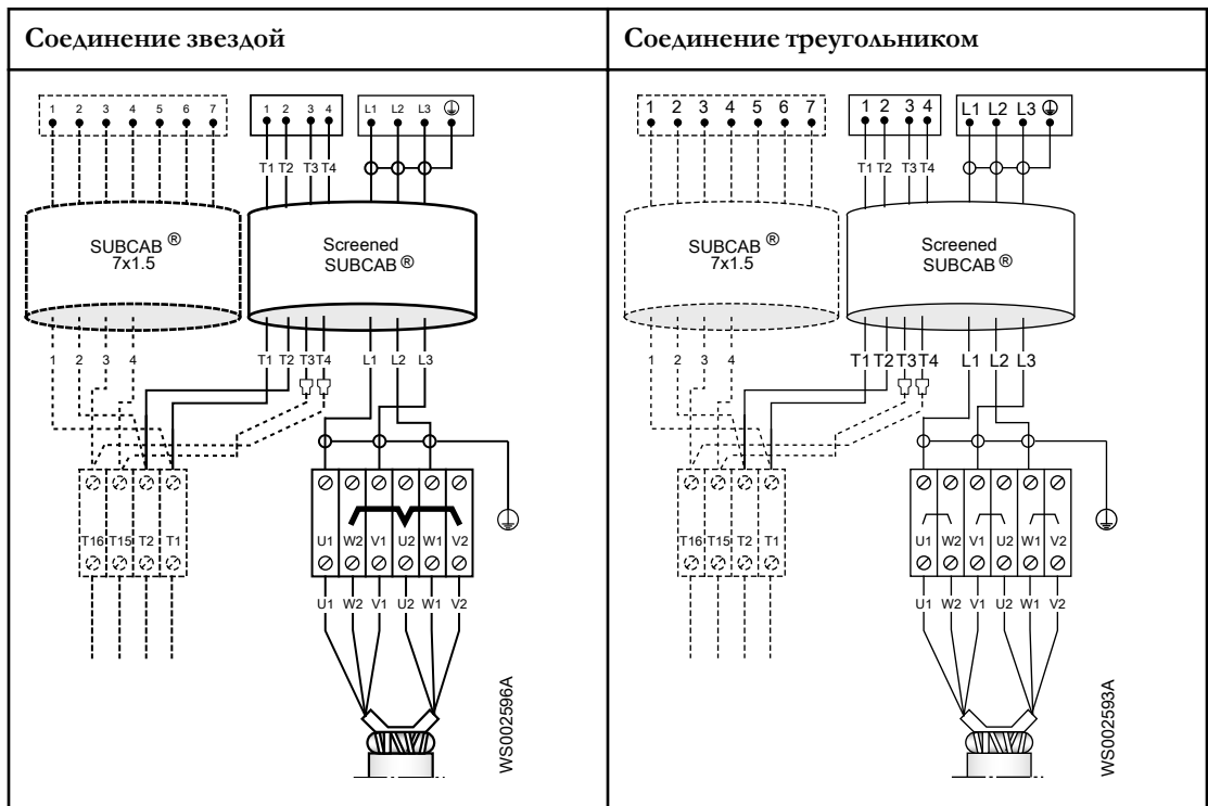
Кабель SUBCAB, экранированный, 6 выводов статора, соединения звездой и треугольником
