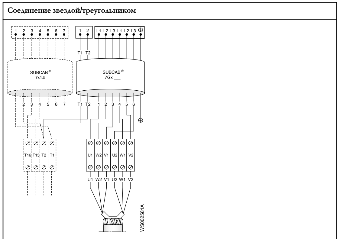
Кабели SUBCAB 4GX / SUBCAB AWG, 6 выводов статора, соединения звездой и треугольником
