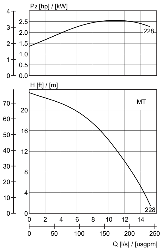
Рис. 18: BS, 3-фазный
