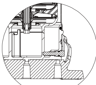
KOREK SPUSTOWY
