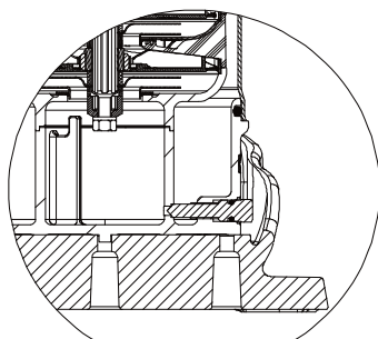
VYPÚŠŤACÍ UZÁVER
