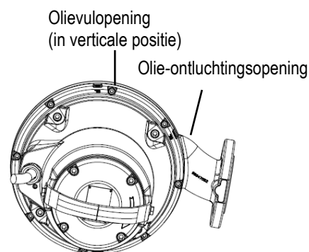
Afb. 11 Olievulopeningen
