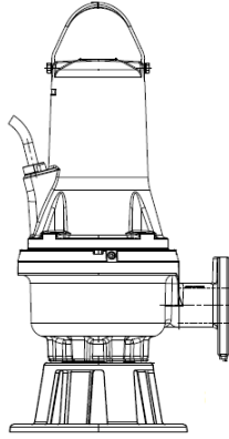
Fig. 7 تركيب مغمرور على قاعدة الدعم
