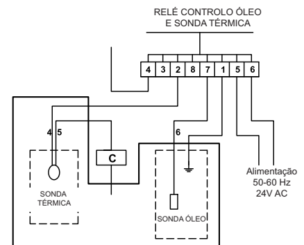
Fig. 13 Ligação da sonda térmica
