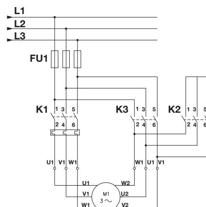
Fig. 11 Conexiuni stea-triunghiulară
