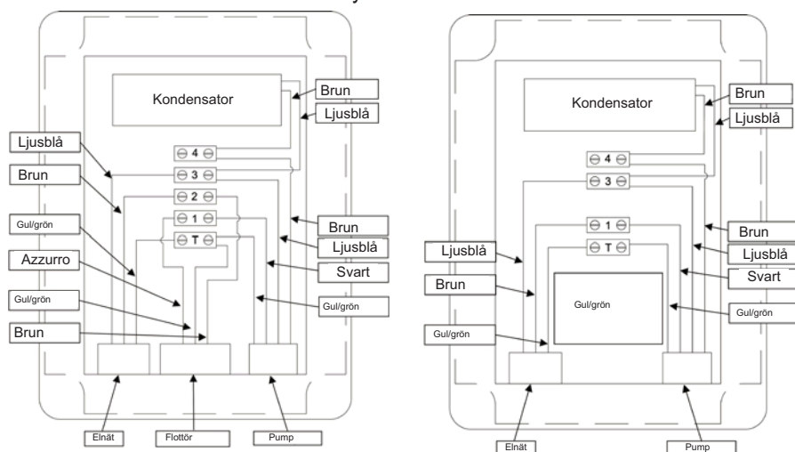
Fig. 8 Kopplingsscheman för en enfaspump med och utan flottör
