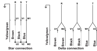
Abb. 10 Dreiphasenanschluss für direkten Anlass
