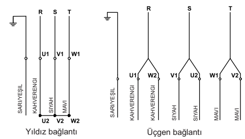
Res. 10 Doğrudan çalışmaya başlatma için trifaze bağlantılar
