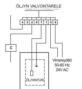
Kuva 14 Tasoanturin liitäntä
