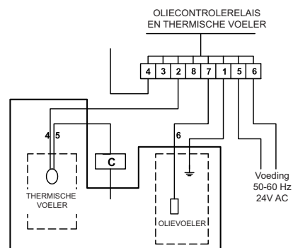
Afb. 10 Aansluiting niveauvoeler
