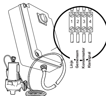
Fig. 9 Eltavla för lågspäningspumpar
