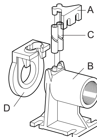
Obr. 7 Spojovací noha
