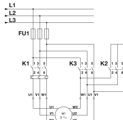
Fig. 11 Ligações estrela-triângulo
