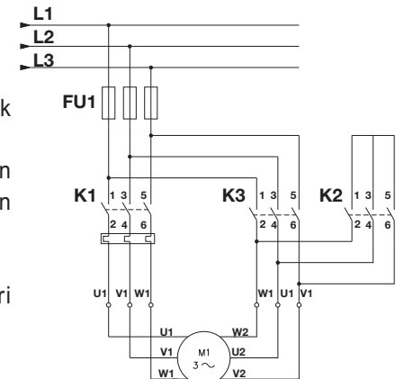
Res. 11 Üçgen yıldız bağlantılar
