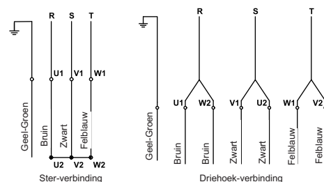
Afb. 10 Driefasige aansluiting voor directe start
