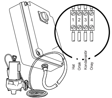
Res. 9 Alçak gerilimli pompalar için elektrik paneli
