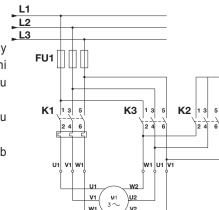
Rys. 11 Połączenie gwiazda-trójkąt
