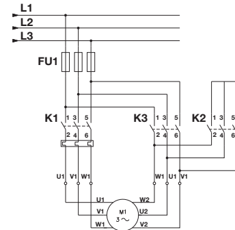
Abb. 11 Anschluss-Schema für den Dreikantstern-Anlass
