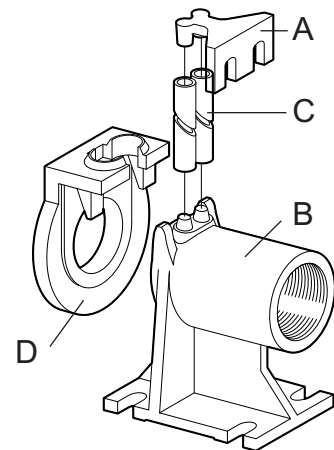
Kuva 7 Kytentäjäjalka
