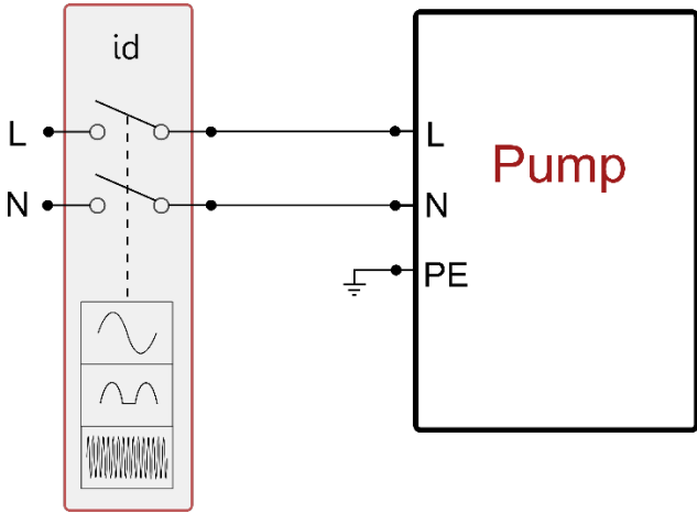
Figure 11 exemple d'installation monophasée
