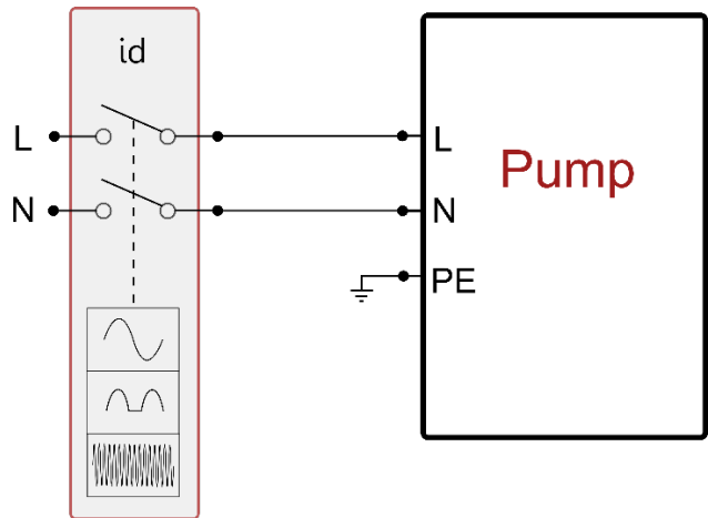
Fig. 11 exemplo de instalação monofásica
