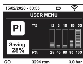
Figura 17 Visualización del histograma de la potencia
