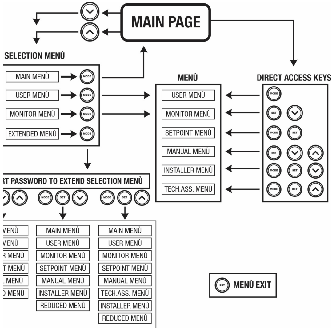
الشكل 13 رسم تخطيطي لإمكانية الوصول إلى القوائم
