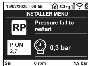
Kuva 18: Uudelleenkäynnistysarvo asetus
