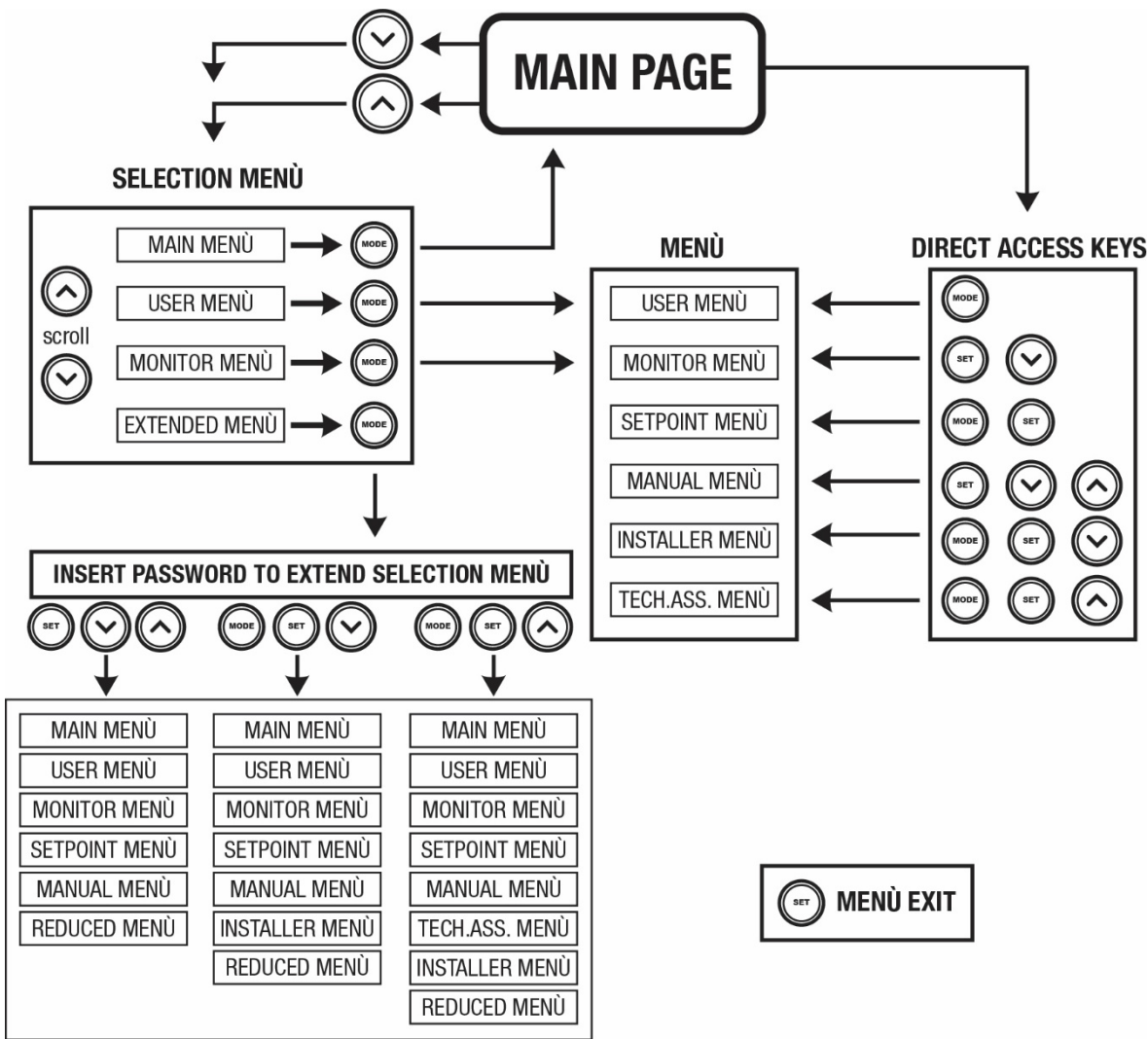
Figura 15: Esquema dos acessos possíveis aos menus
