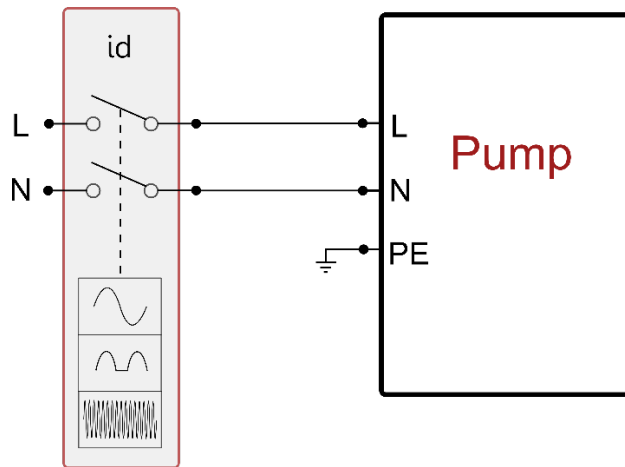
Εικ.11 παράδειγμα μονοφασικής εγκατάστασης
