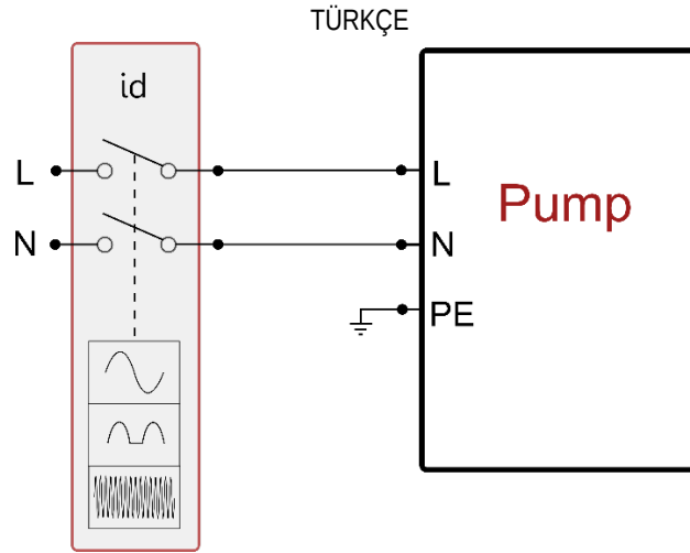
Şekil 11 monofaze kurulum örneği
