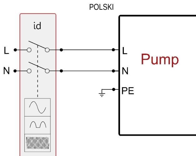
Rys. 11 przykład instalacji jednofazowej
