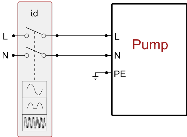
Рис. 11 пример однофазной установки
