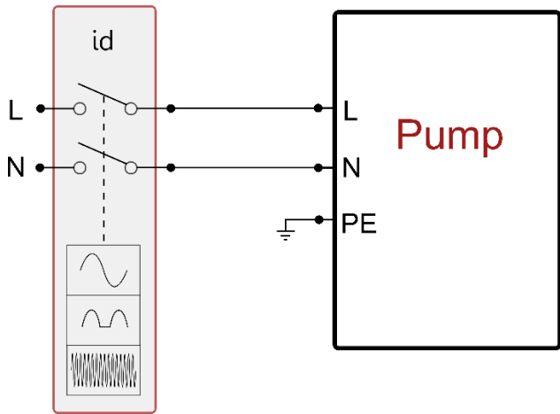
Fig 11 esempio di installazione monofase
