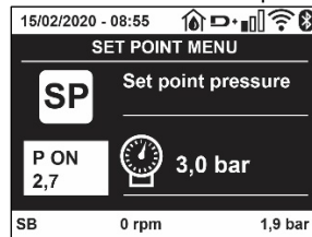
Kuva 16 Valikkoparametr
