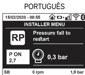
Figura 18: Programação da pressão de rearmar
