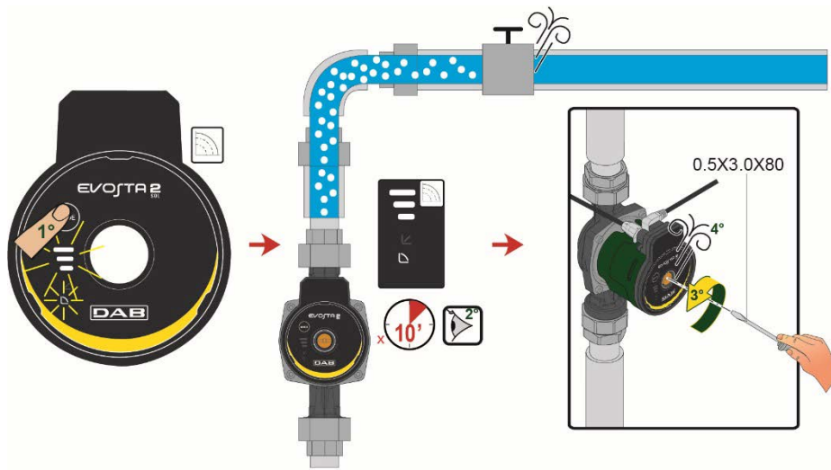
Abb 16: Pumpenentlüftung
