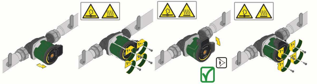
Фигура 14: Промяна на позицията на потребителския интерфейс
