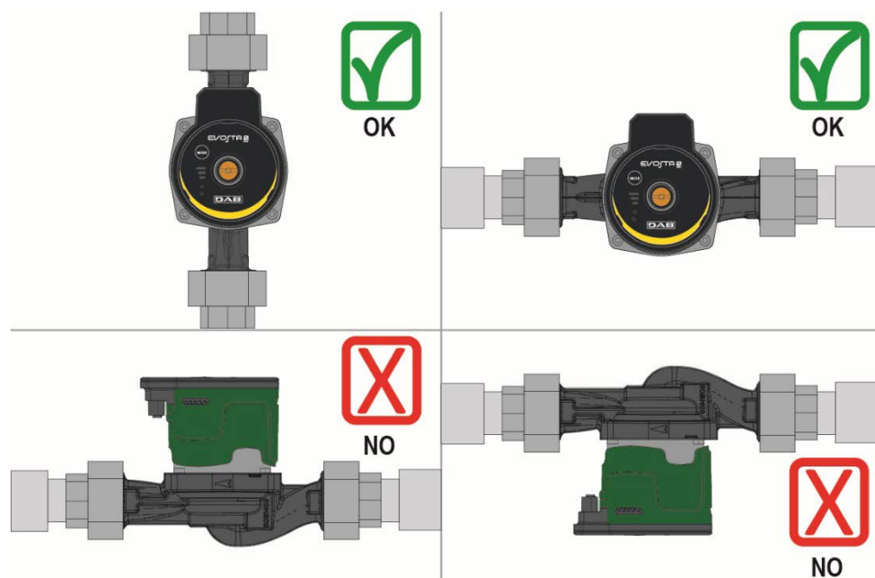
Slika 12: Vgradni položaji
