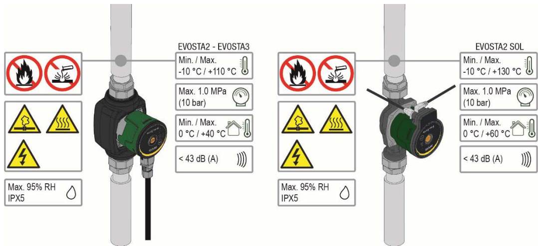
Figura 1: Líquidos bombeados, avisos e condições de funcionamento
