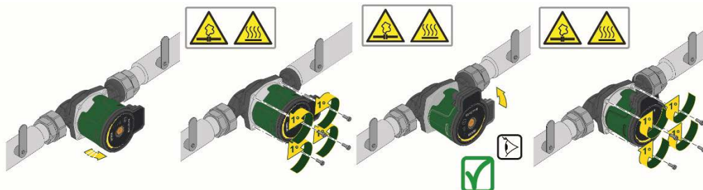
Рисунок 14: Изменение положения пользовательского интерфейса
