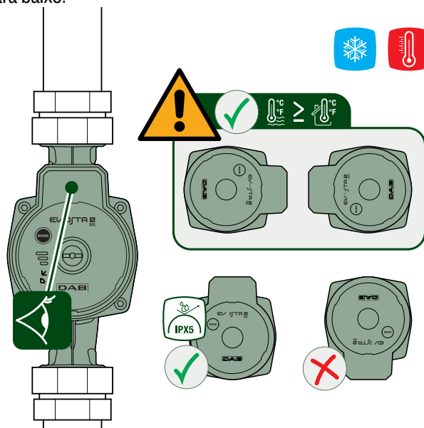
Figura 4: Posições da interface utilizador
