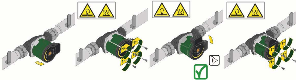
Kuva 14: Käyttöliittymän asennon muutos
