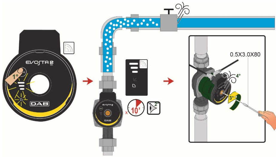
Kuva 16: Pumpun ilmaus
