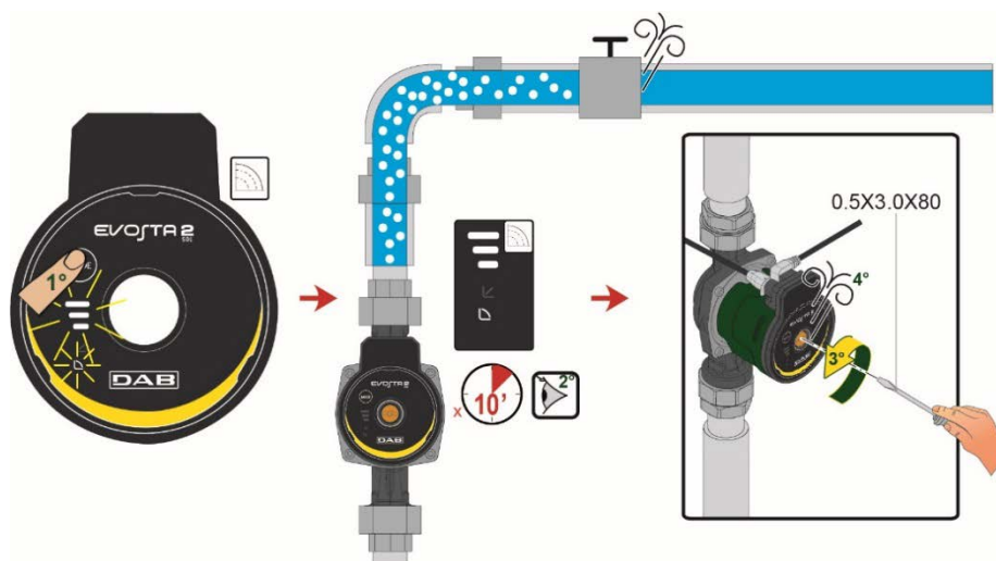
16. ábra: Pumpa légmentesítés
