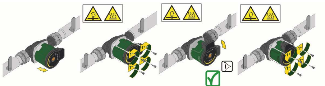
Slika 14: Sprememba položaja uporabniškega vmesnika
