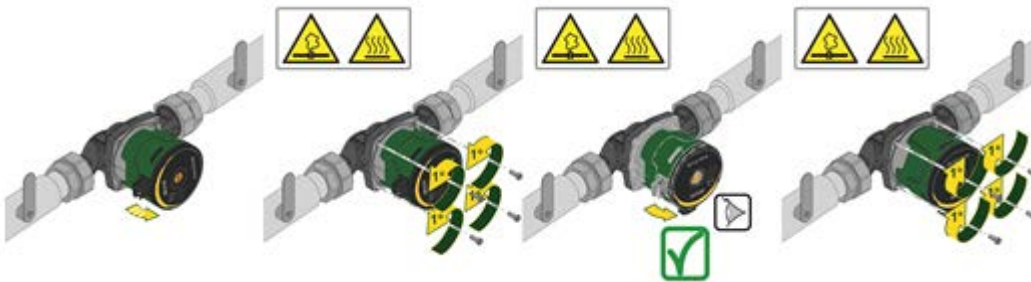
Kuva 5: Käyttöliittymän asennon muutos
