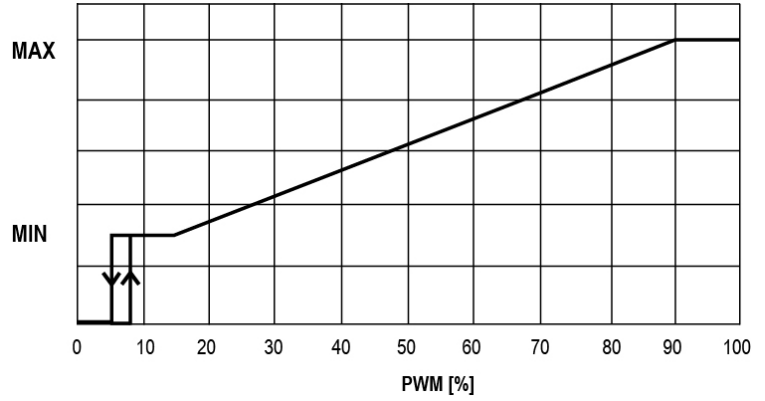
GÜNEŞ PWM Profili
