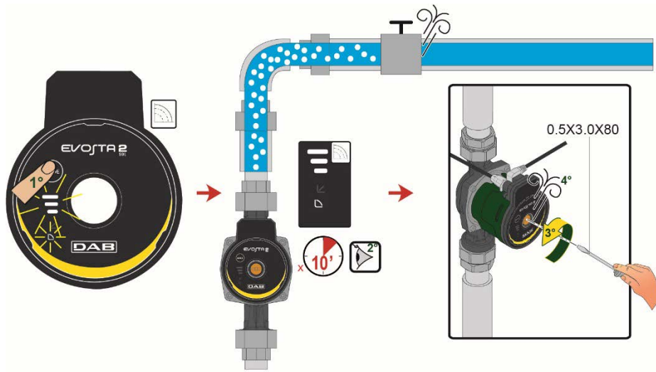
Obrázok 16: Odvzdušnenie čerpadla
