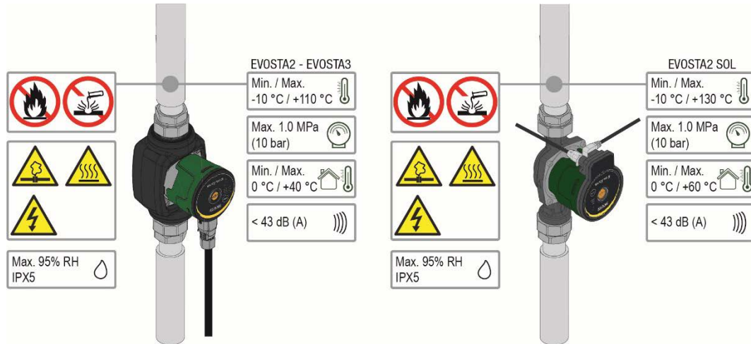
الشكل 1 : ضخ السوائل، والتحذيرات، وظروف التشغيل
