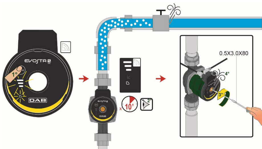
Obrázek 16: Odvzdušnění čerpadla
