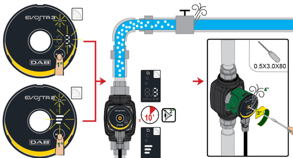
Obrázok 7: Odvzdušnenie čerpadla
