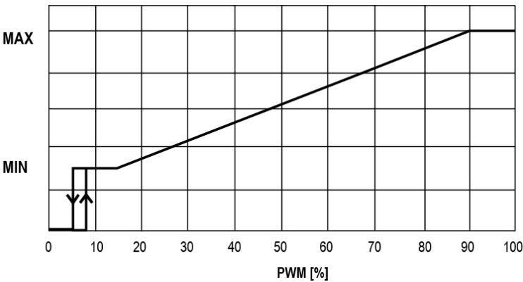
Perfil PWM SOLAR
