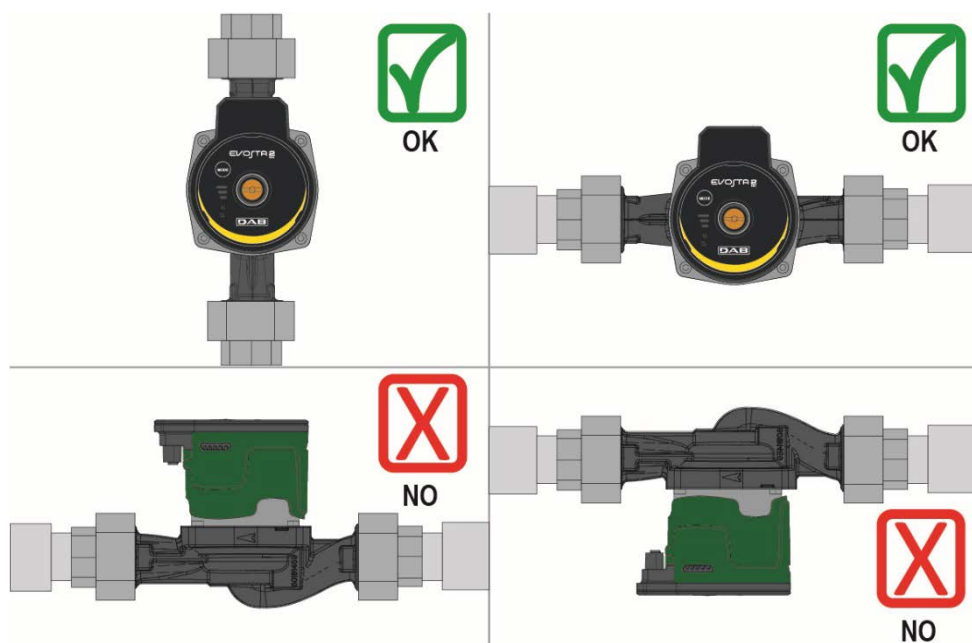
Fig 12: Monteringsläge
