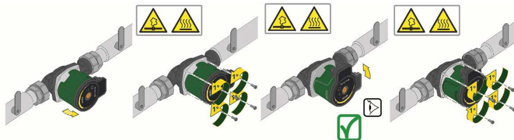
Obrázek 14: Změna polohy uživatelského rozhraní
