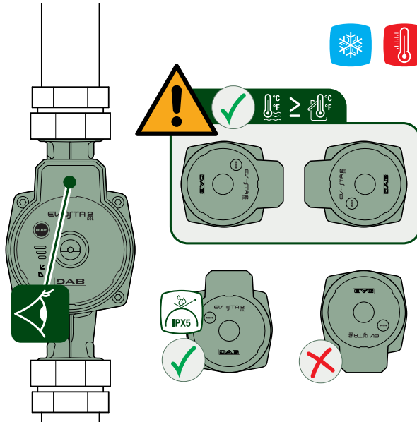
الشكل 13: مواضع واجهة المستخدم
