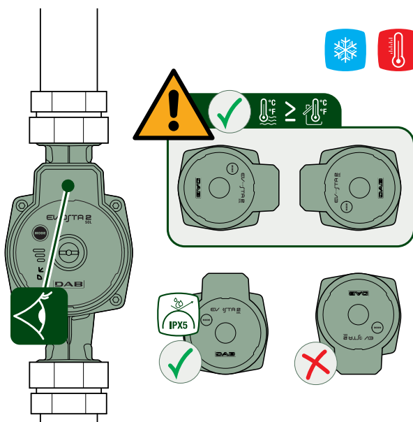
Obrázek 13: Poloha uživatelského rozhraní
