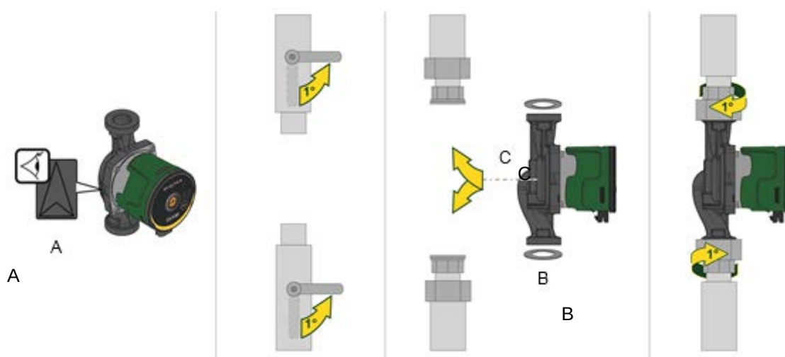
Fig. 2: Monterings af EVOSTA2 eller EVOSTA3
