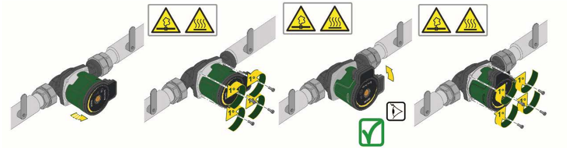
Fig 14: Ändring av användargränssnittets position
