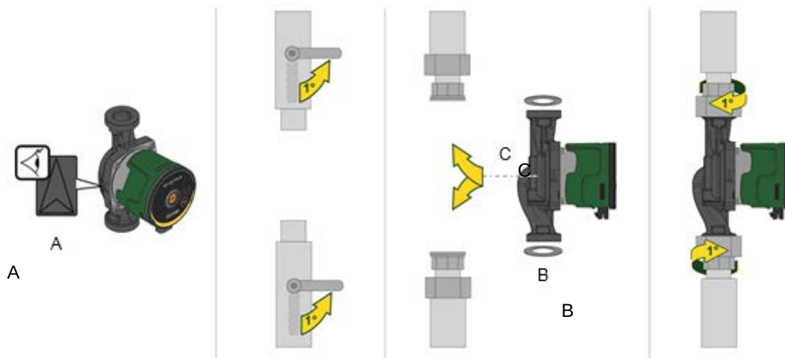
Fig 2: Monteringsdiagram för EVOSTA2 eller EVOSTA3
