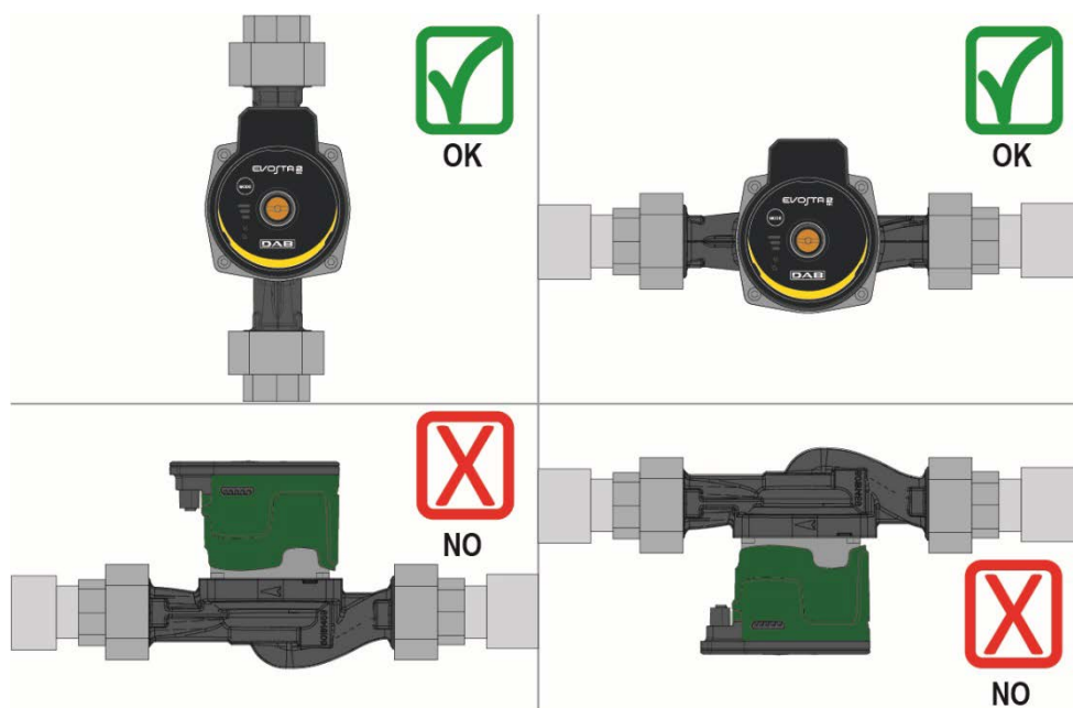
Kuva 12: Asennusasento
