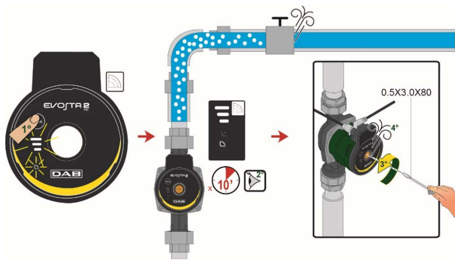
Slika 16: Odzračitev črpalke
