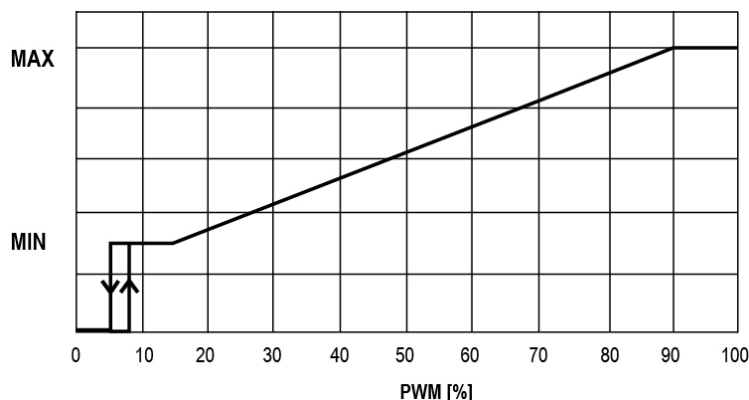
PWM-profil SOL
