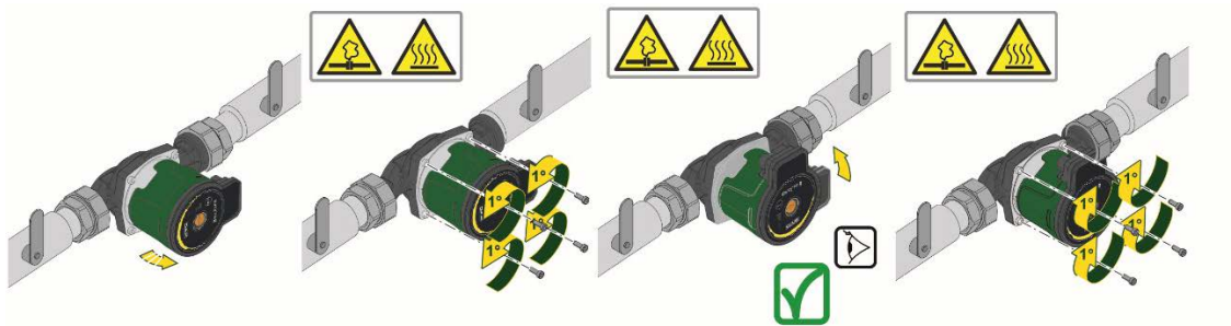
Figura 14: Cambio de la posición de la interfaz del usuario
