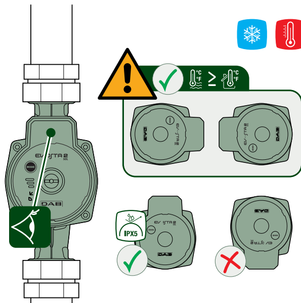
Figura 13: Posizioni dell'interfaccia utente
