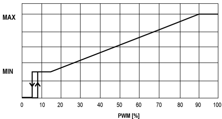
Προφίλ PWM SOLAR
