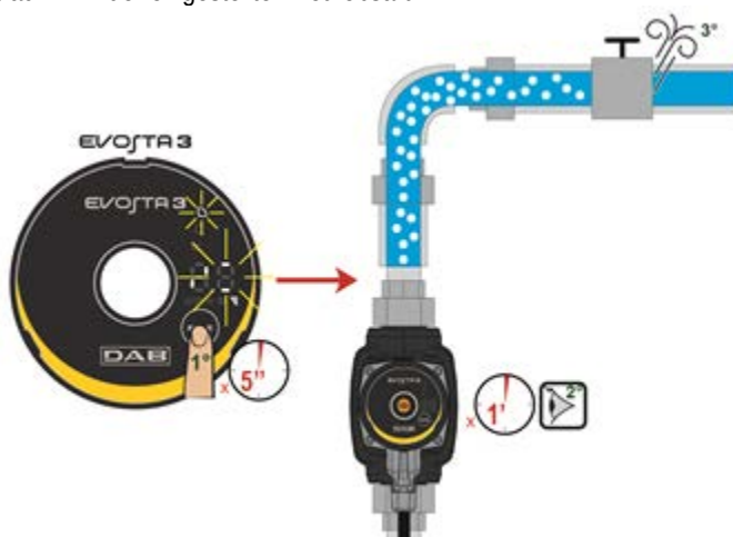
Abb. 8: Automatische Pumpenentlüftung
