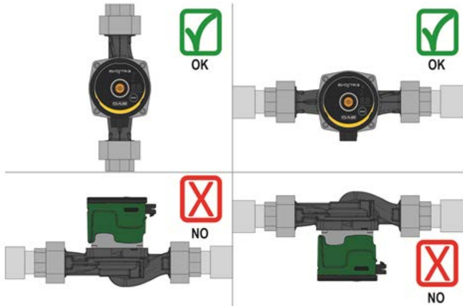
Resim 3: Montaj pozisyonu
