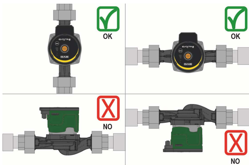
Obrázok 12: Montážna poloha
