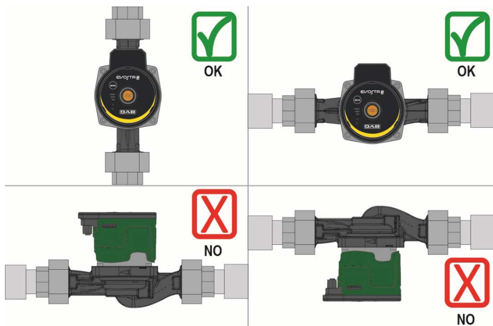
Fig. 12: Monteringsposition
