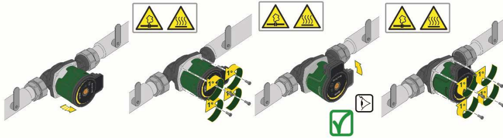
الشكل 14: تغيير موضع واجهة المستخدم
