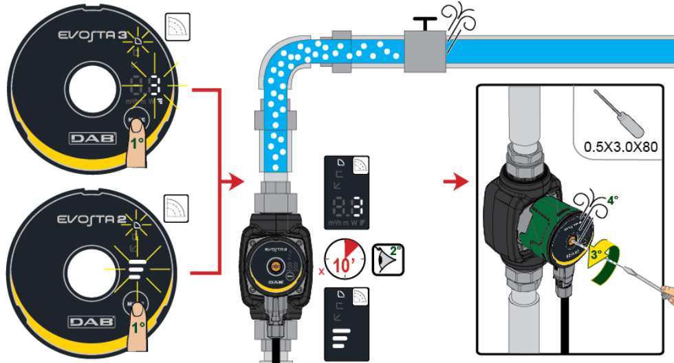
الشكل 7: تنفيس المضخة
