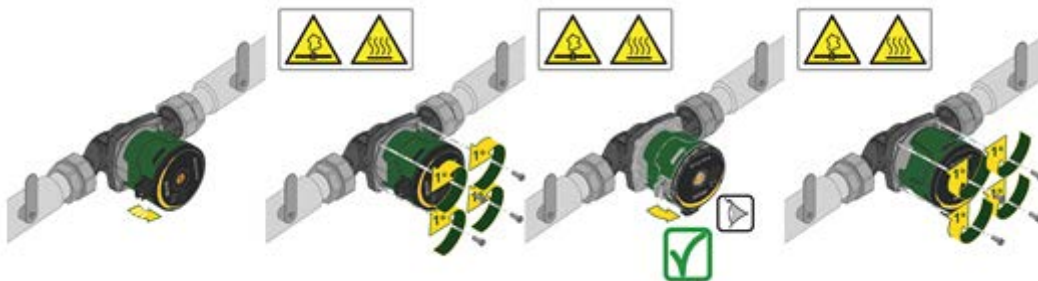
5 pav.: Vartotojo sąsajos padėties keitimas
