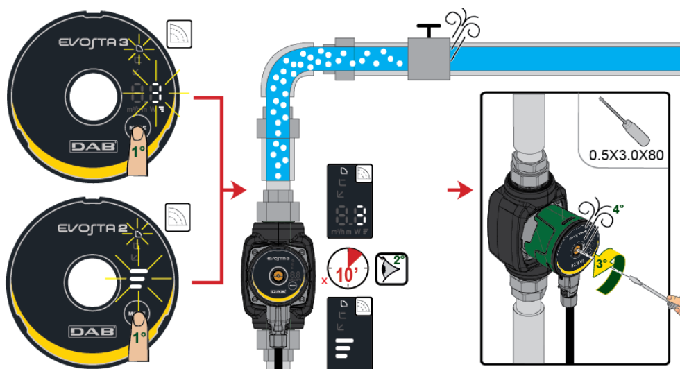
Kuva 7: Pumpun ilmaus
