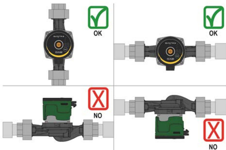
Afbeelding 3: montagepositie
