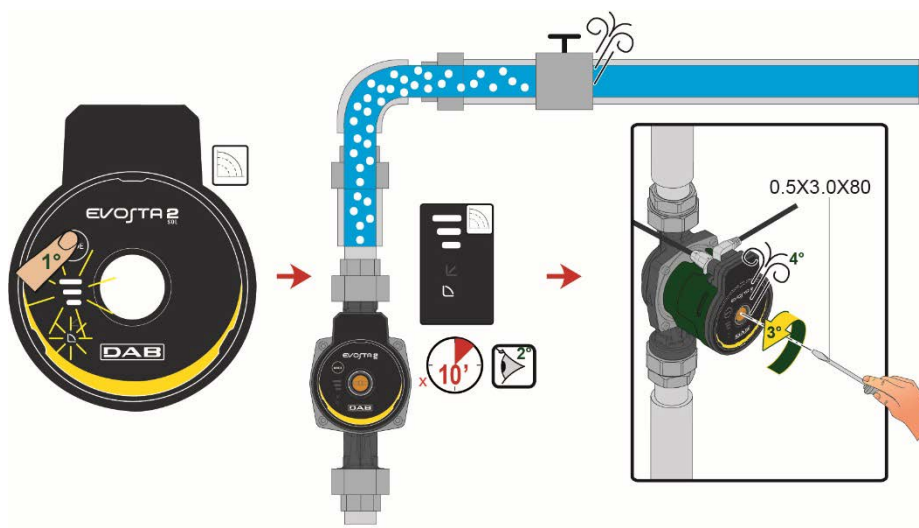
Figura 16: Aerisirea pompei
