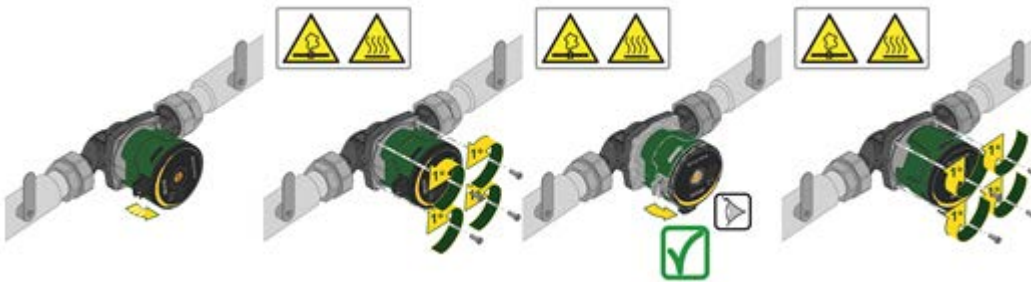
Obrázok 5: Zmena pozície užívateľského rozhrania
