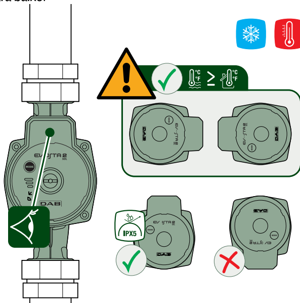
Figura 13: Posições da interface utilizador
