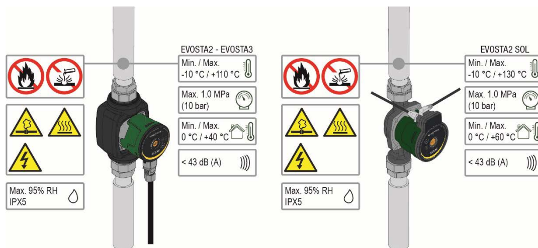
Fig 1: Vätskor, varningar och driftsförhållanden
