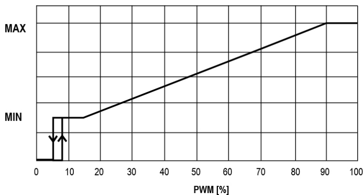
PWM-profil SOL
