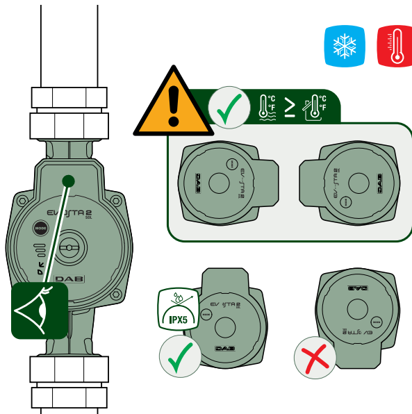
13 pav.: Vartotojo sąsajos padėtys
