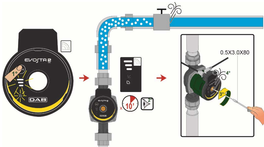
Attēls 16: Sūkņa gaisa izvadīšana
