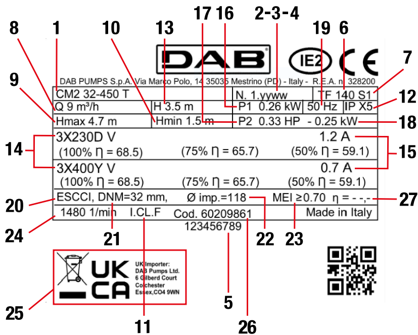
Fig.1 Etiqueta
