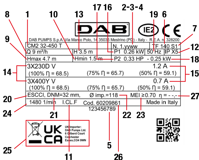
Fig.1 Targhetta
