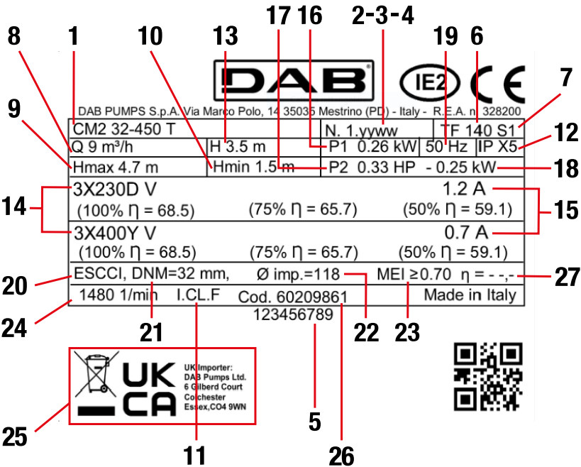
Abb. 1 Typenschild
