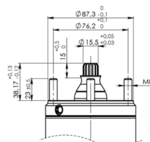
NEMA FLANGE
