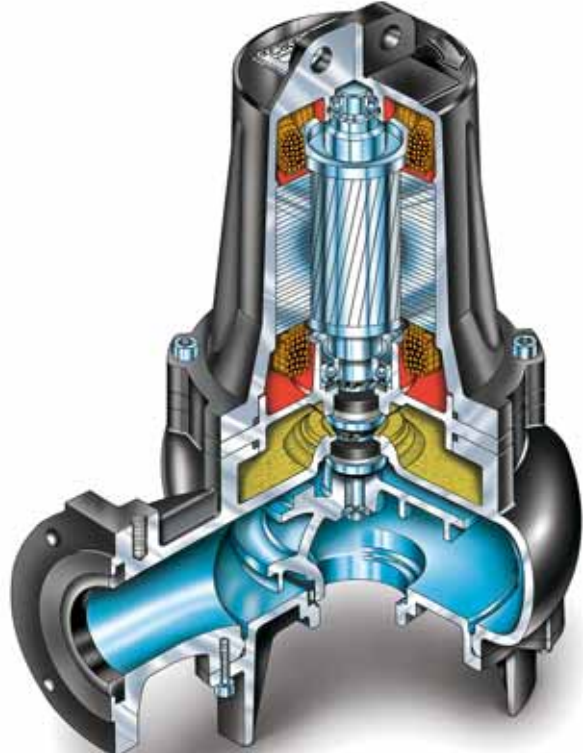
Girante-Impeller-Roue
