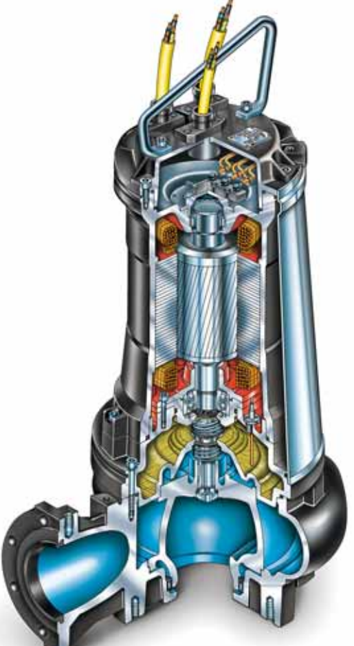
Girante-Impeller-Roue
