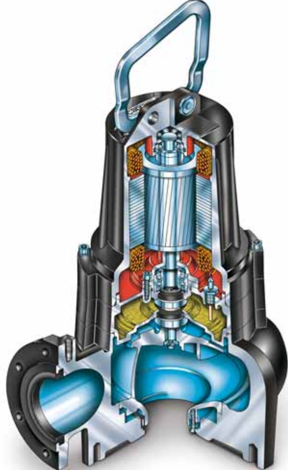
Girante-Impeller-Roue
