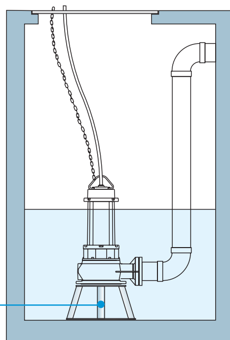
Embase en fonte sphéroïdale Base de fundición esferoidal
