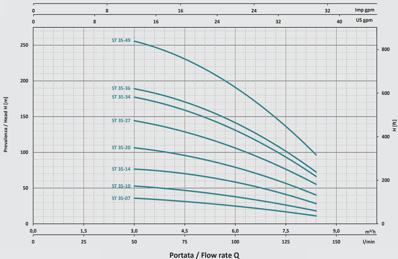
Prestazioni / Performance Data 50Hz
