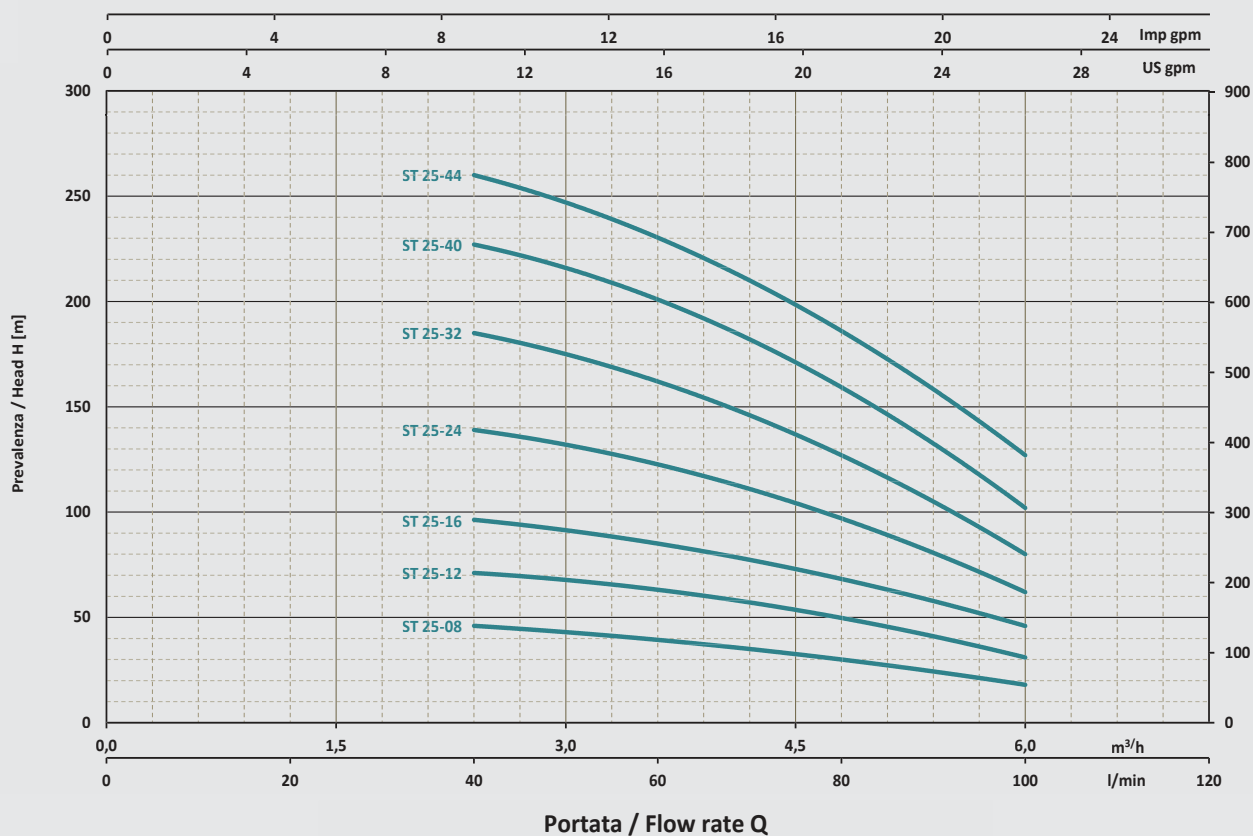
Prestazioni / Performance Data 50Hz
