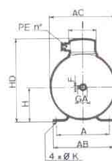
FIXATION PAR SOCLE
