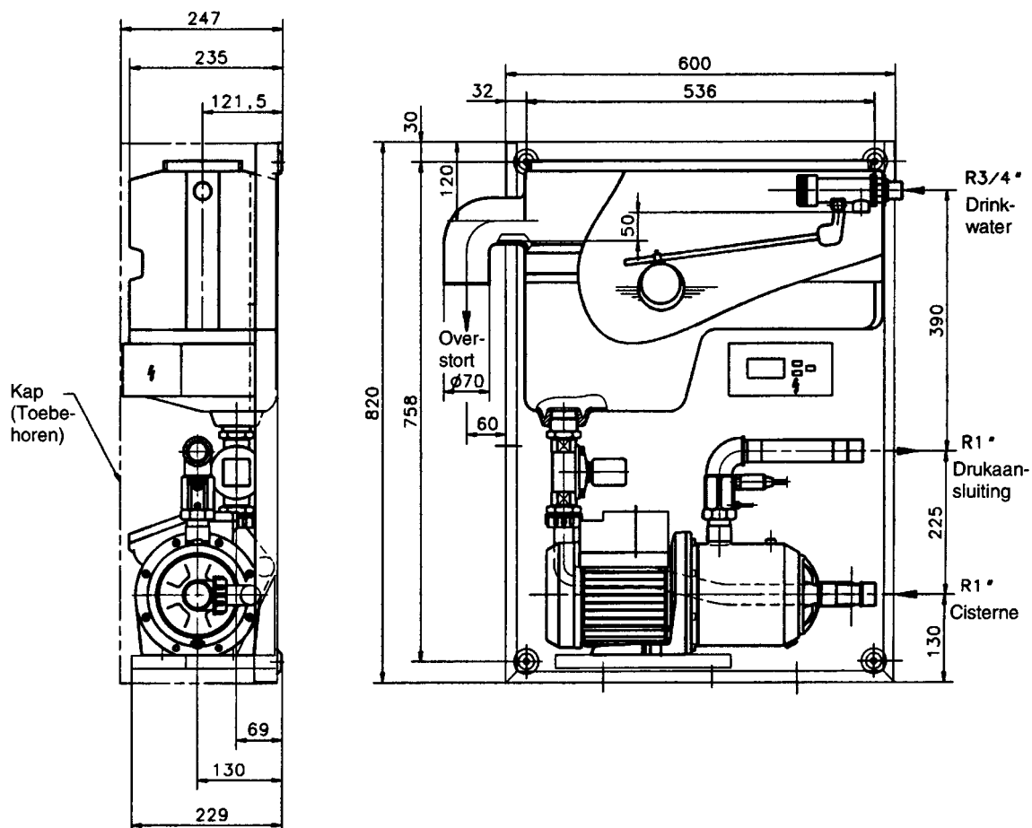
Figuur 5. Schema met hydraulische aansluitingen
