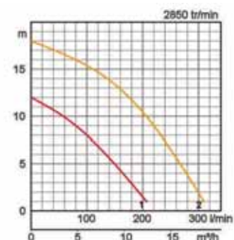
Pompe d'épuisement équipée d'un corps de type spirale.
