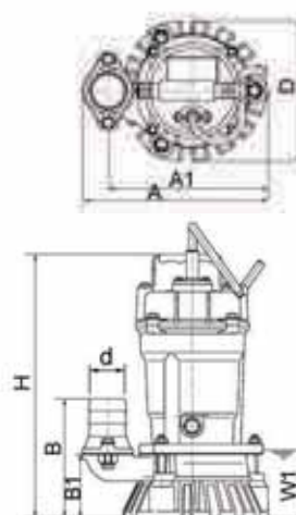
W1: Niveau minimum de pompage
