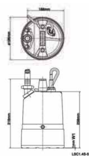
W1: Niveau minimum de pompage
