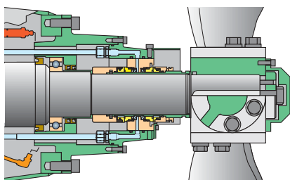
Garniture mécanique simple ou double
