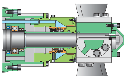
Garniture mécanique simple protégée
