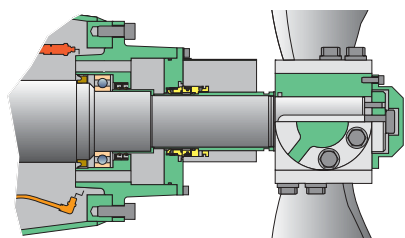
Garniture mécanique simple ou double
