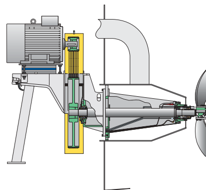
Pieds supports et Dilco pour eau de dilution
