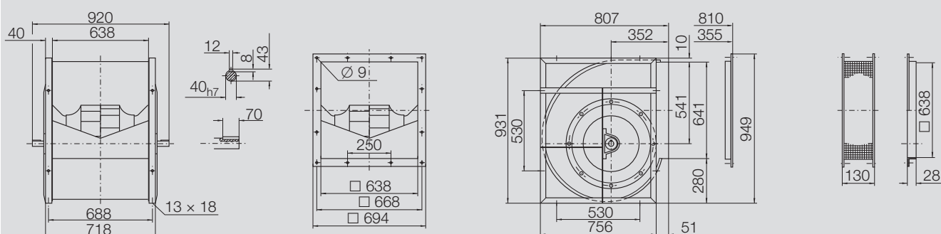
RDH E6-0500 92 kg
