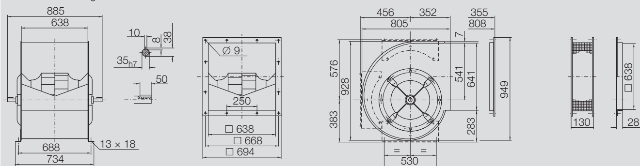
RDH E2-0500 70 kg
