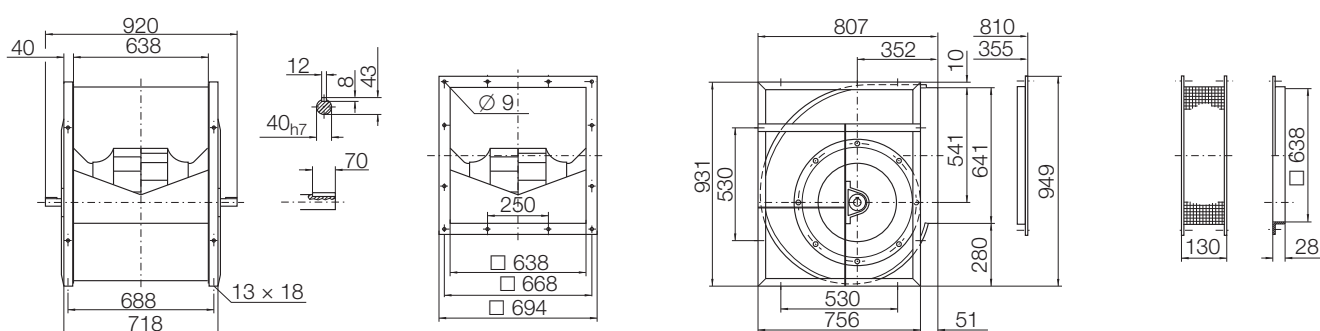
RDH E7-0500 110 kg
