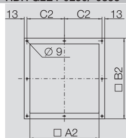
RDH G2E4-0250/-0560 / RDH G2K-0630/-1000
