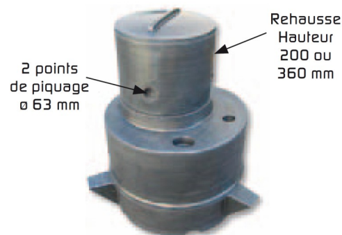
Poste de relevage 250 litres avec rehausse
