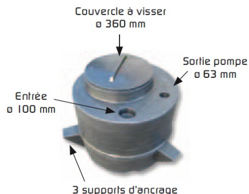
Poste de relevage 250 litres
