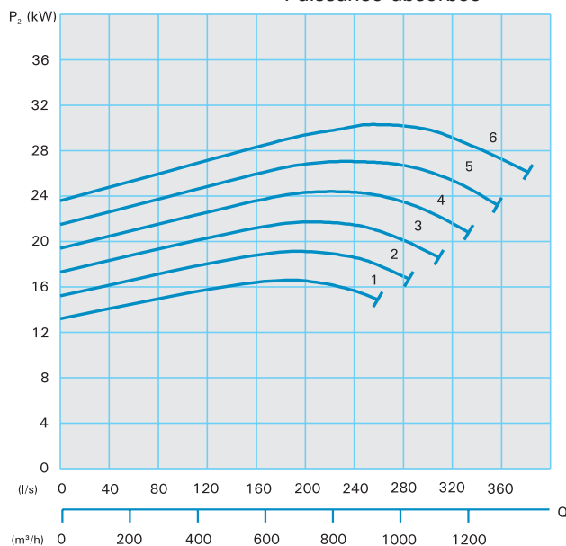
Puissance absorbée
