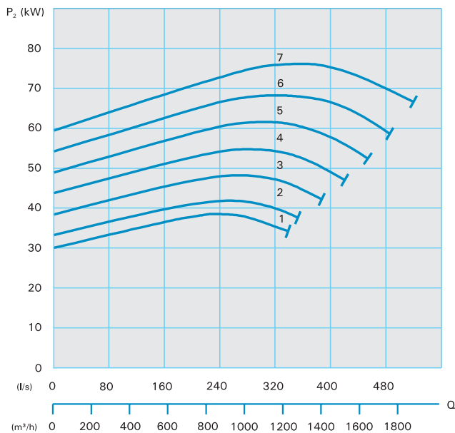
Puissance absorbée
