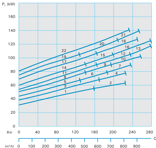
Puissance absorbée
