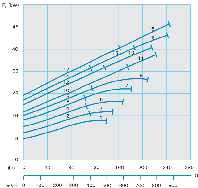
Puissance absorbée
