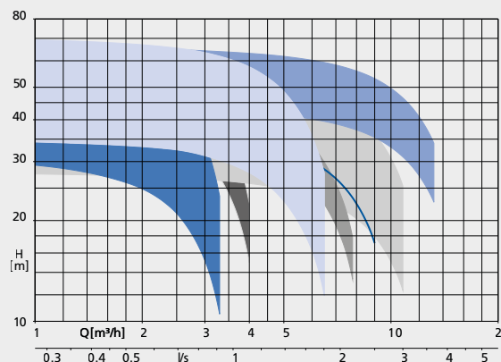
Courbes caractéristiques - 1 pompe
