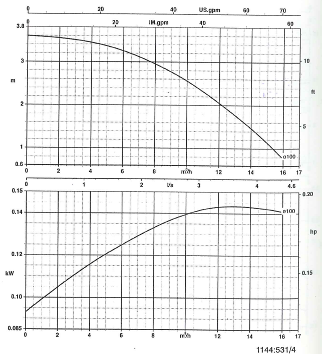
Trialine Z 50-125/024
