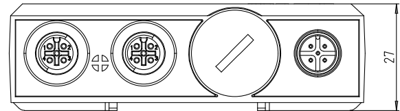
III. 3: Dimensions du capteur, plage de mesure à partir de 65 bar
